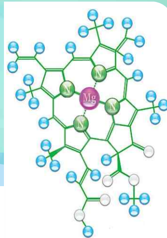
Molécula de clorofila
